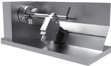
Fix megtámasztás vég megmunkáláshoz
