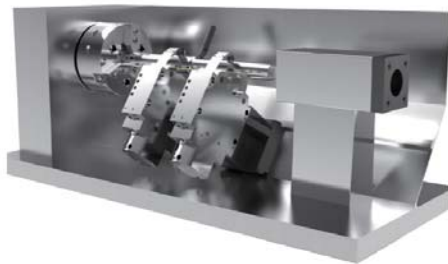
Kettős fix támasztás
