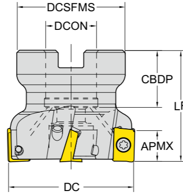
2 élű lapka
